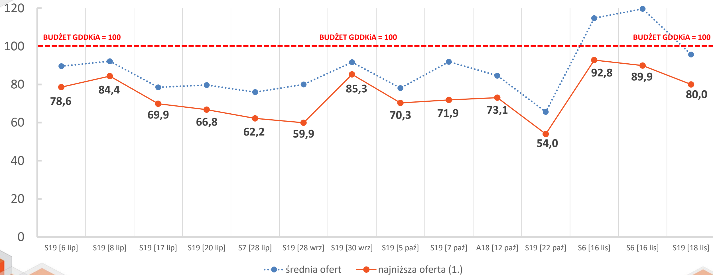
Wykres 6. Oferty generalnych wykonawców na tle kosztorysów GDDKiA [w %]
